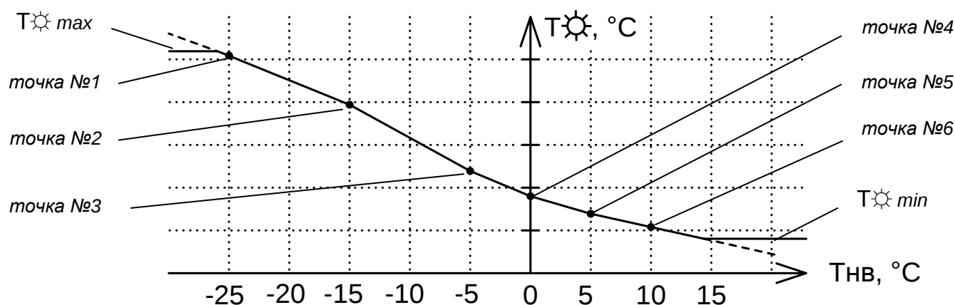
Рисунок 15 - Температурный график
