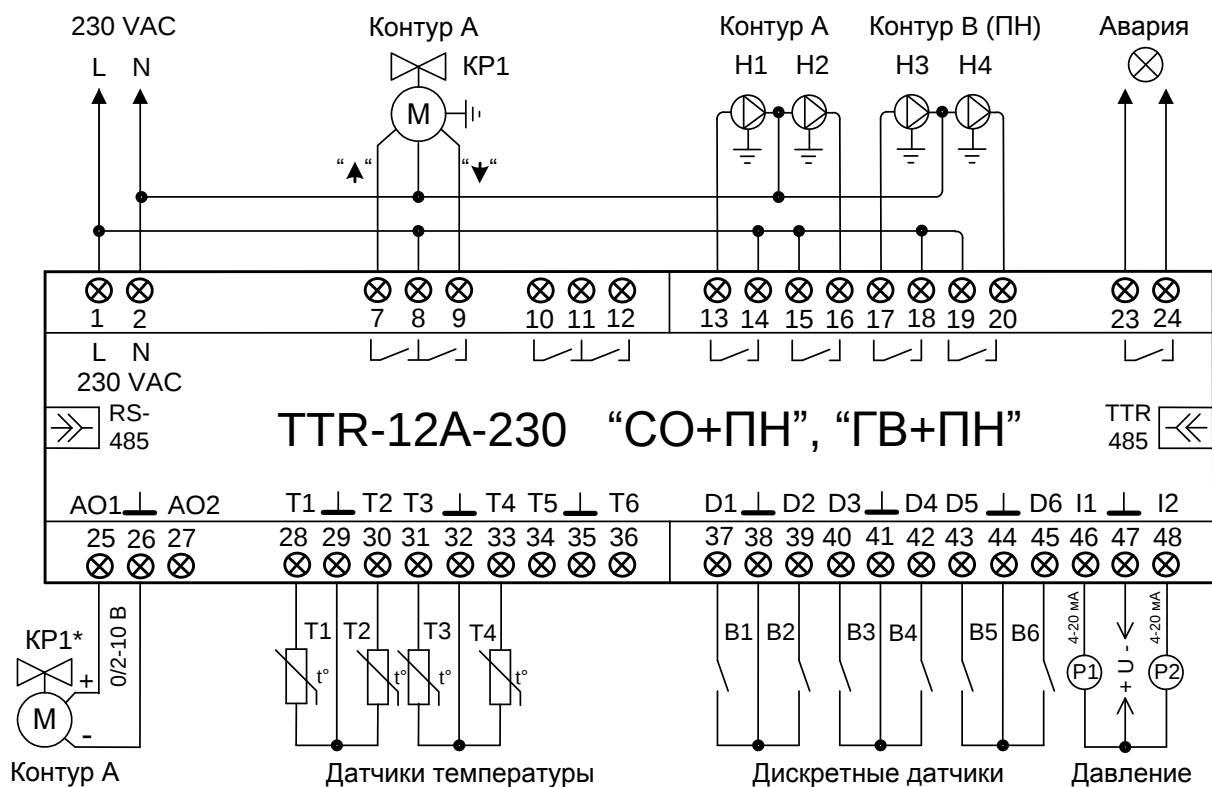
Рисунок В.4 – Схема подключений ТТR-12А-230 для одноконтурной СО или ГВС с дополнительным контуром повысительных насосов (ПН)
