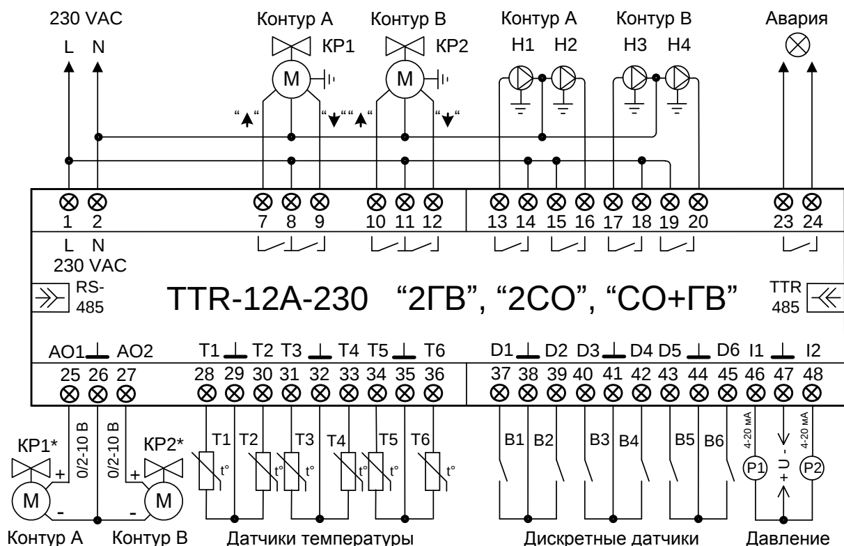
Рисунок В.3 – Схема подключений ТТR-12А-230 для двухконтурной СО и ГВС
