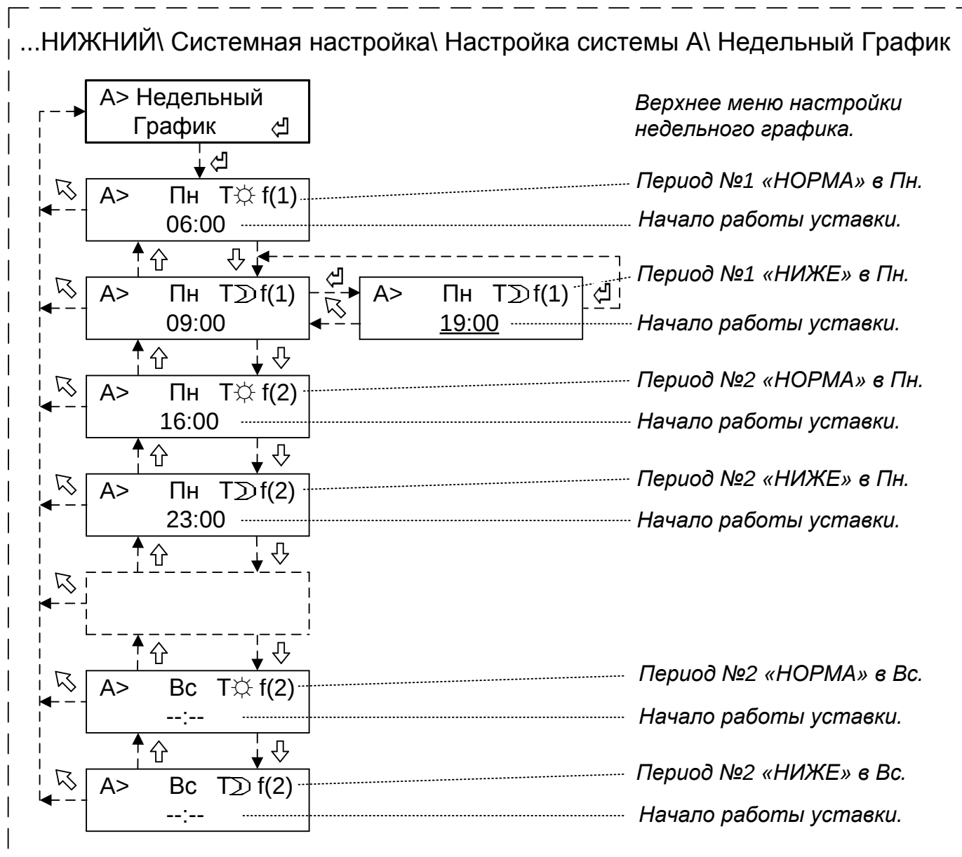
Рисунок 18 - Структура меню настройки временного (недельного) графика
