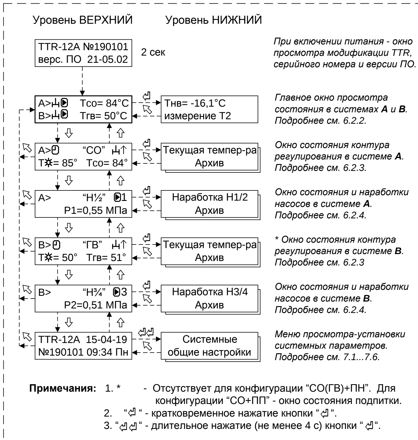
Рисунок 3 – Общая структура пользовательского меню
