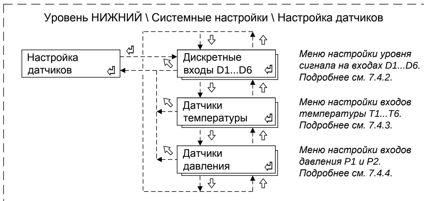
Рисунок 7 – Структура меню настройки входов и выходов
