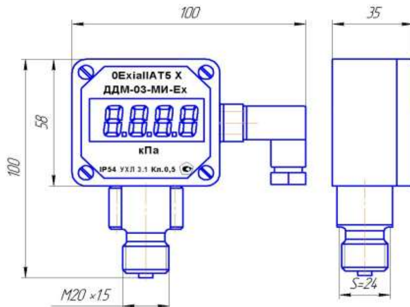
Рис.1. Габаритные и присоединительные размеры датчиков ДДМ-03-xx-ДИ-МИ-Ех
