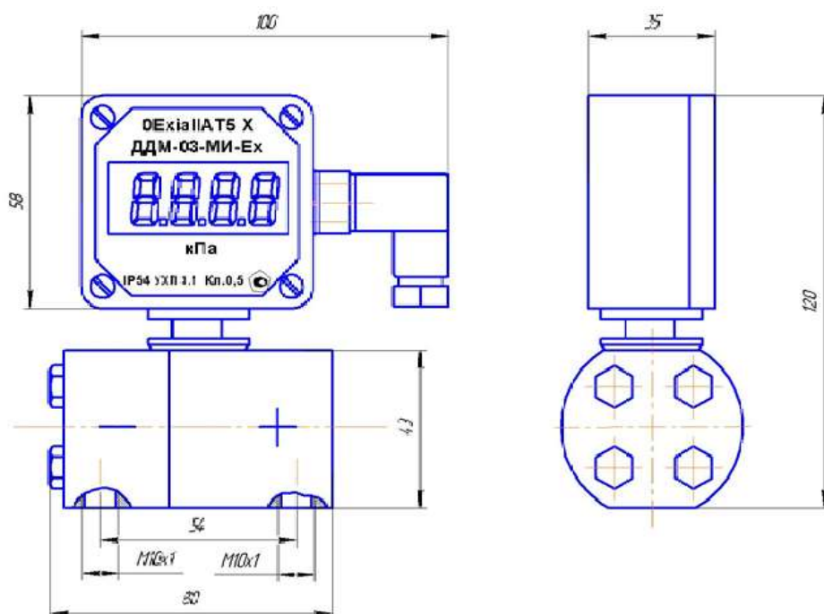
Рис.2. Габаритные и присоединительные размеры датчика ДДМ-03-ДД-МИ-Ex
