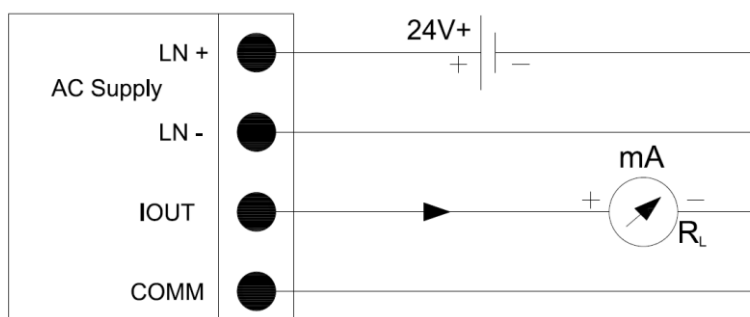
Токовый выход - четырехпроводное соединение (гальванически развязан)
