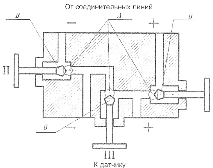
Рисунок 1 — Схема клапанного блока
