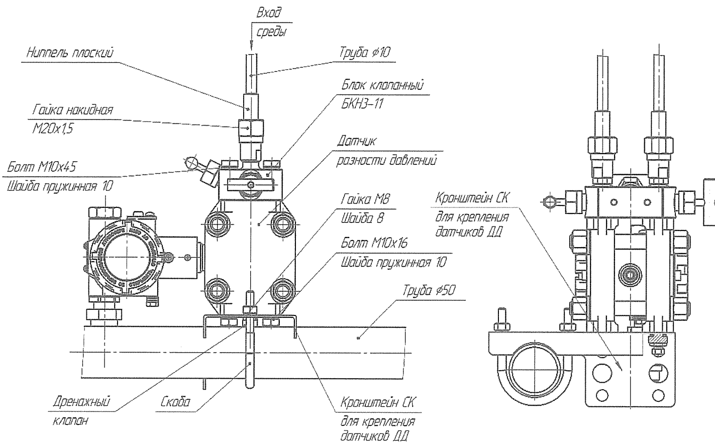
Рисунок Л1.3 - Монтажный чертеж установки преобразователя давления фланцевого конструктивного исполнения с смонтированным клапанным блоком "БКН" резьбового присоединения к импульсным линиям, и с КМЧ "Фланец М20" и "Кронштейн СК" (для крепления датчиков ДД). Вариант крепления на горизонтальной трубе \phi 50
