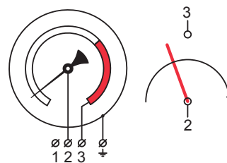
Положение стрелки Состояние контакта
