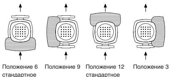
Рис. 33 Положение клеммной коробки
