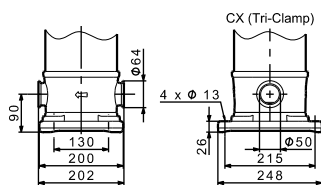
FGJ (DIN-ANSI-JIS), PN 16-25 / DN 50
