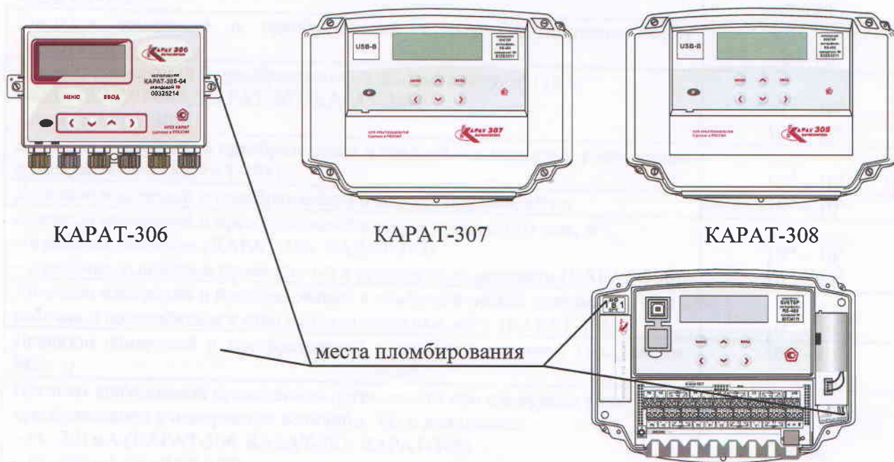
Рисунок 1 – Внешний вид и места пломбирования вычислителей
