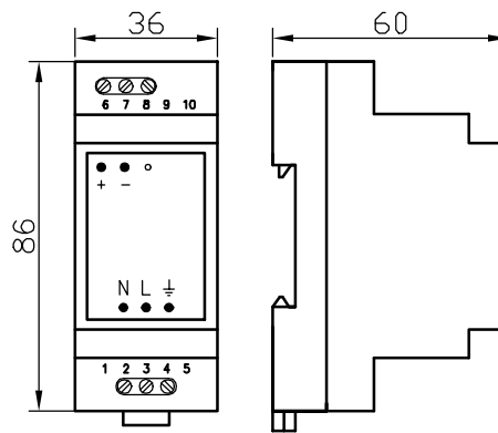
Рис. 1 - Габаритный чертёж
