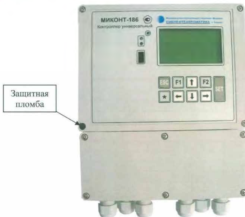
Рисунок 6 - Схема пломбировки контроллера МИКОНТ-186 от несанкционированного доступа
