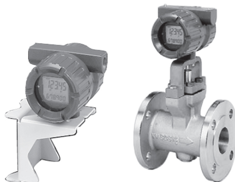
Вихревой преобразователь (разнесенного типа)
