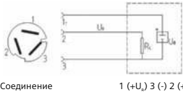
Соединение 1 (+U 0 ) 3 (-) 2 (+U 0 )
