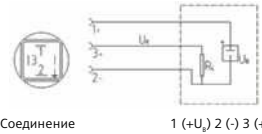
Соединение 1 (+U 0 ) 2 (-) 3 (+U 0 )
