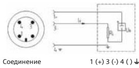
Соединение 1 (+) 3 (-) 4 (-) ↓
