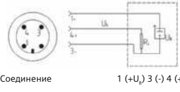
Соединение 1 (+U 0 ) 3 (-) 4 (+U 0 )
