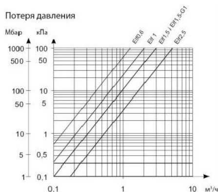
Рисунок 1. Потери давления на проточной части теплосчётчика.
