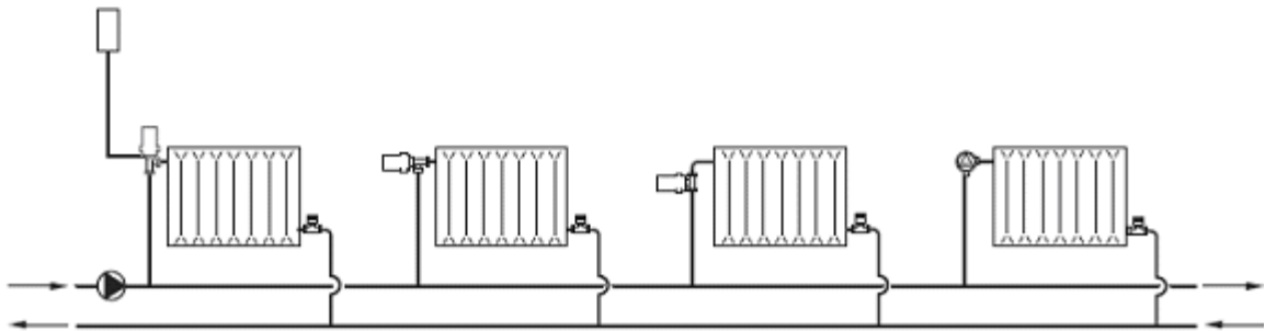
Рис.2 Двухтрубная насосная система отопления
