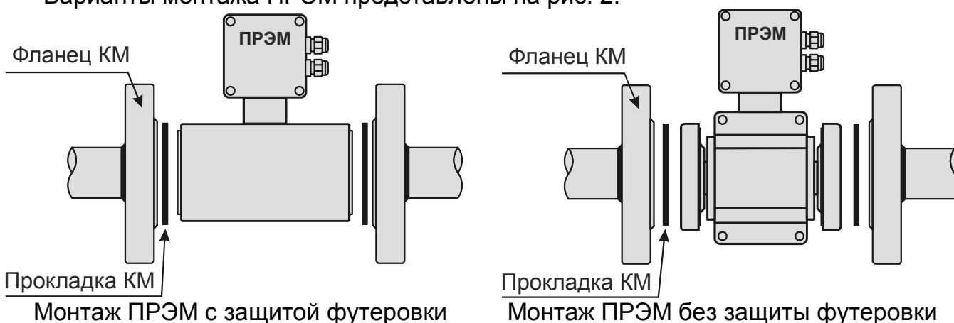
Рисунок 2 – Варианты монтажа ПРЭМ
