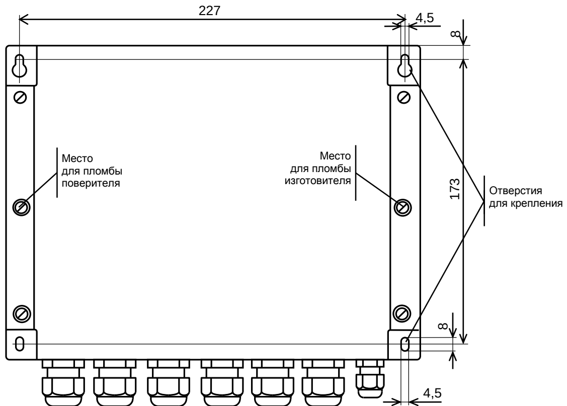
Рисунок 3.3 – Вид сзади
