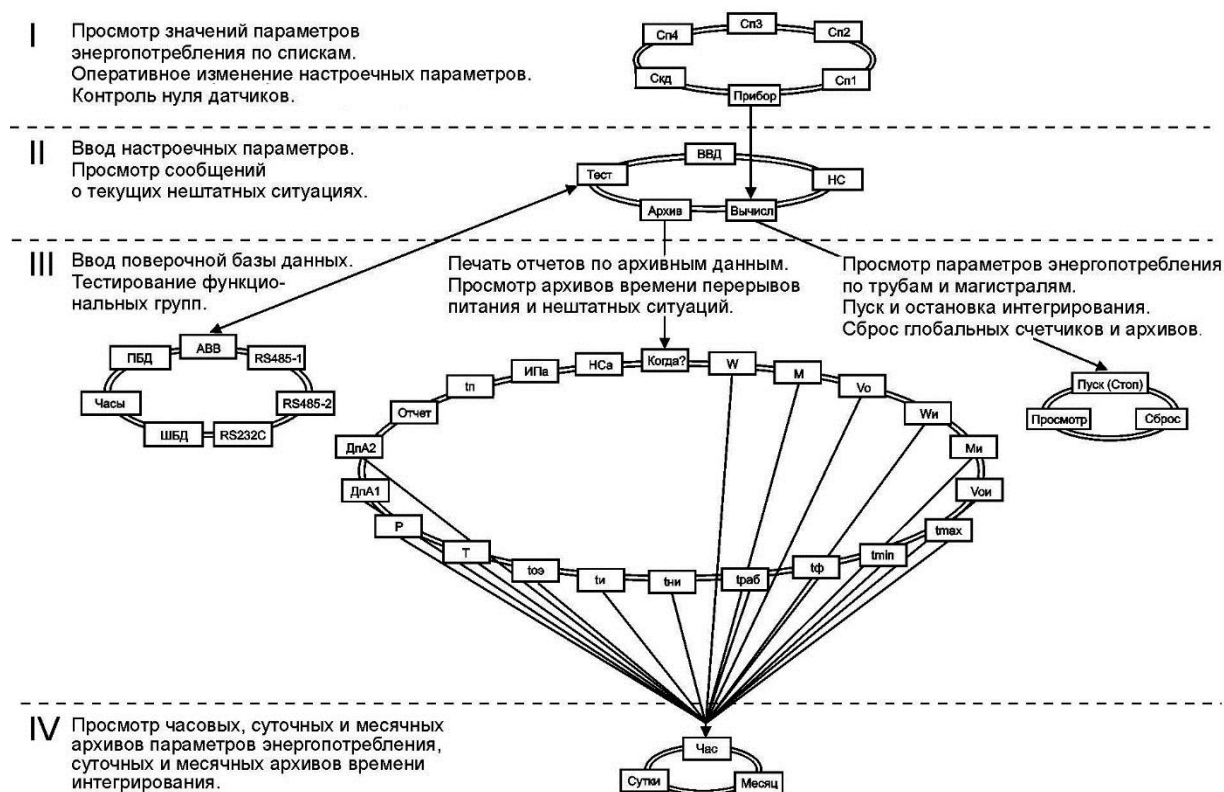
Рисунок 6.1 – Структура меню
