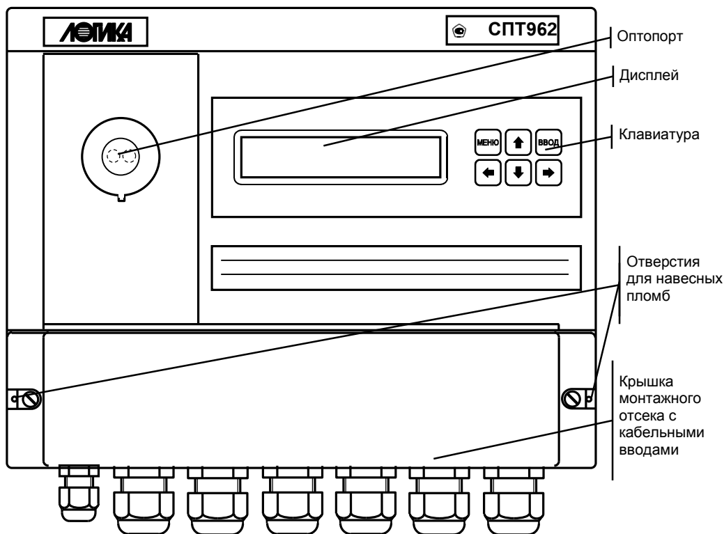
Рисунок 3.1 – Вид спереди
