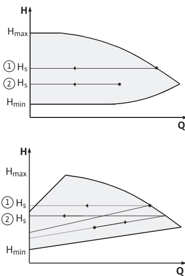
Рис. 40: Регулирование Др-с/Др-в
