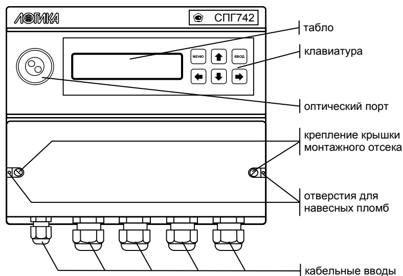
Рисунок 3.1 – Вид спереди
