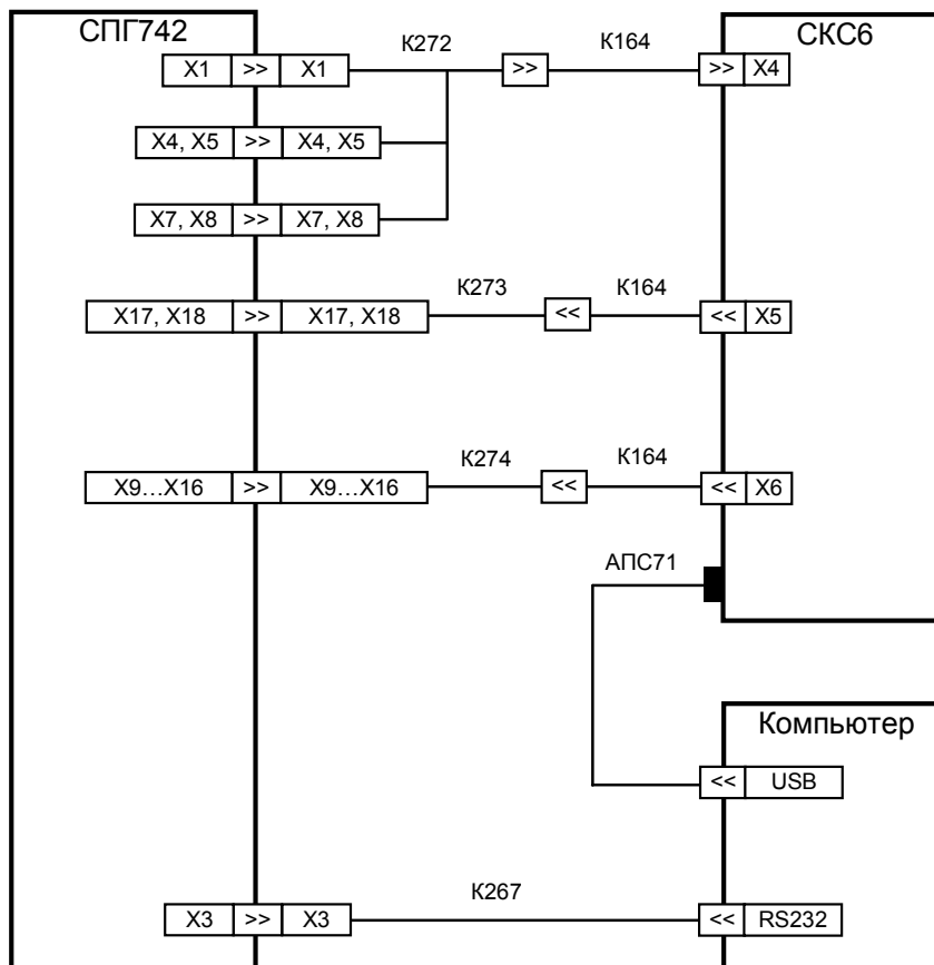
Рисунок 11.1 – Схема проверки
