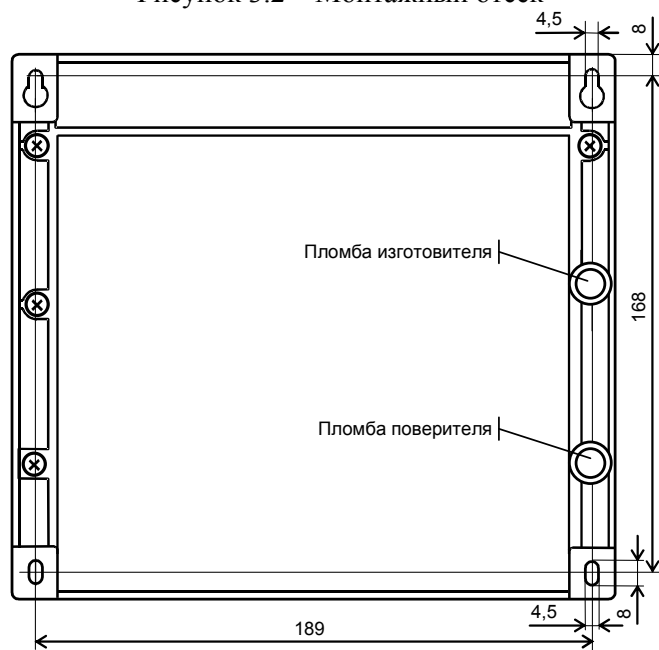
Рисунок 3.2 – Монтажный отсек
