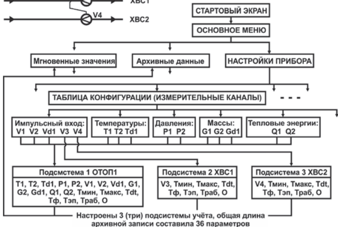
Рисунок 2.5 – Пример реализации алгоритма настройки вычислителя
