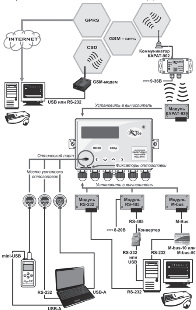
Рисунок 1.3 – Коммуникационные возможности вычислителя
