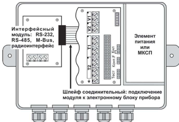
Рисунок Б.4 – Внешний вид монтажного отсека вычислителя KAPAT-306 с установленным интерфейсным модулем
