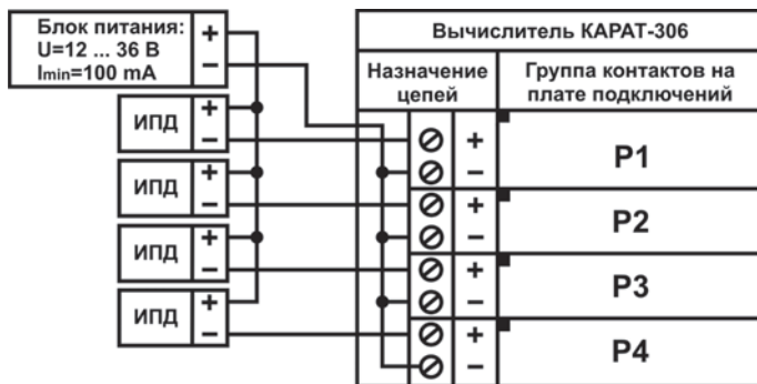
Рисунок В.1 – Схема подключения ИПРВ, ИПРГ, ВС и СВЧ
