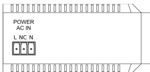
Рис.9. Разъём POWER AC IN.
