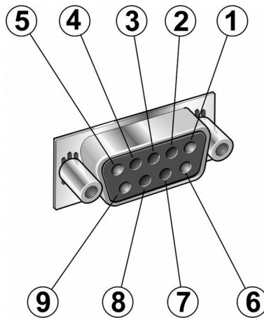
Рис.12. Разъем интерфейса RS-232 (типа D-Sub DB-9F).
